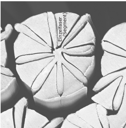
Abb. 7 Elektronen-Mikroskopische Schnittbild-Aufnahme eines einzelnen Matrix-Filaments im Garnstrang des HiTech-Reinigungstuchs Typ MICROWEB®-UDG (Bildbreite 22,4 µm).
