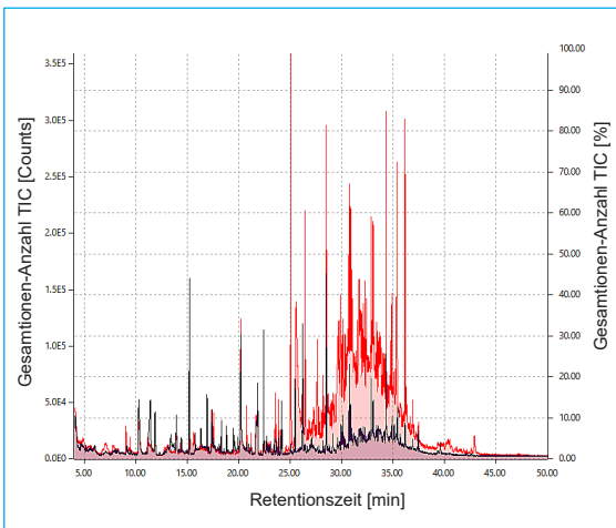
Abb. 8 Reinheits-Prüfung des Cellulosic-Rohmaterials aus China (rot) und Europa (schwarz), Bestimmung mittels GCMS, Beispiel aus unserer QC-Arbeit.
