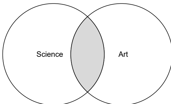
Fig. 20 Diagramme de Venn d'après H. W. Franke Catalogue de l'exposition Microphotographie / La beauté au-delà du visible.
